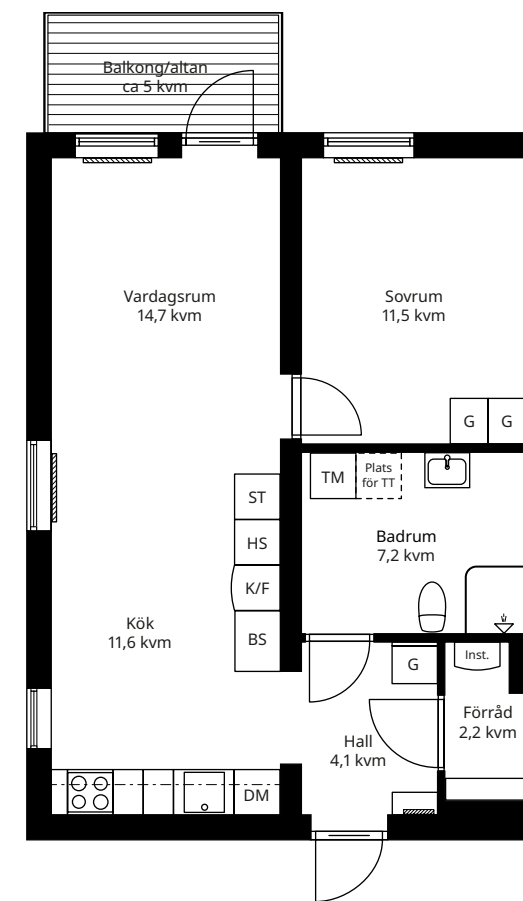
Spiegelvänd planlösning, gavellägenhet, skala 1:100.
