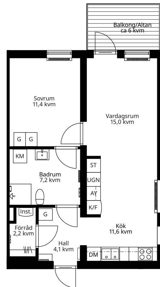
Rätvänd planlösning, gavellägenhet, skala 1:100.
