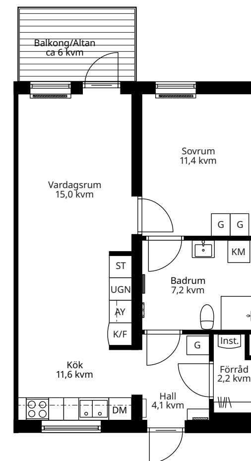
Spiegelvänd planlösning, mittlägenhet, skala 1:100.
